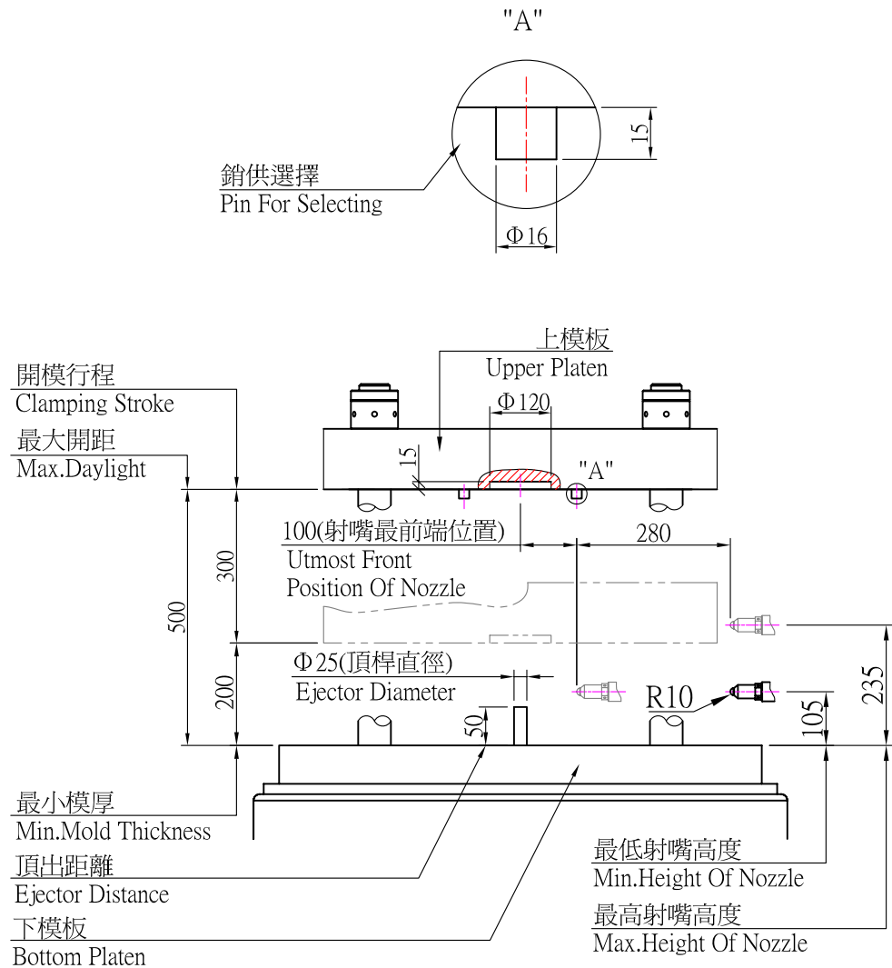
開模規格示意圖(Clamping Unit Diagram)
