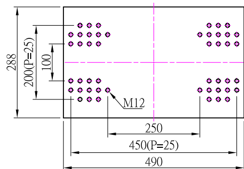
上模板(Upper Platen)
