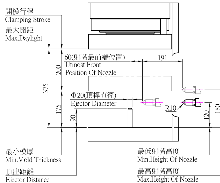
開合模規格示意圖(Clamping Unit Diagram)
