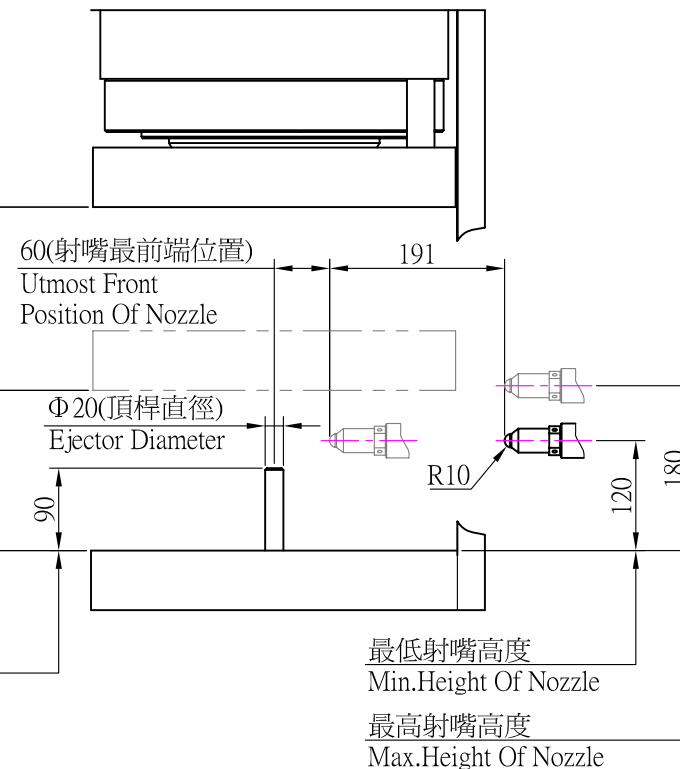
開合模規格示意圖(Clamping Unit Diagram)
